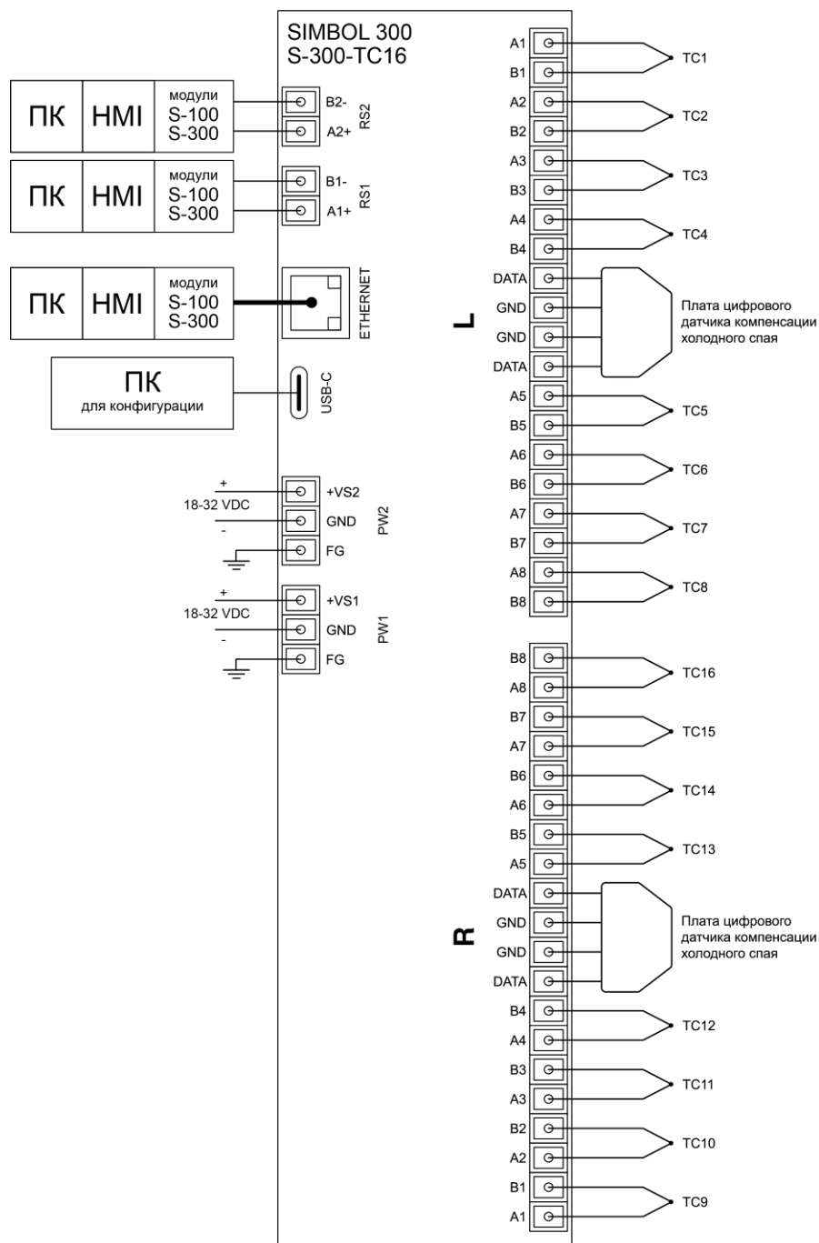
Рисунок 1.5 – Схема подключения модуля контроллера Simbol-300 S-300- TC16 (S-300-TC8)
