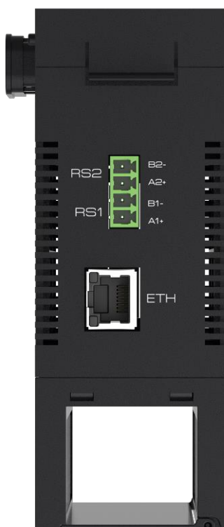
Рисунок 1.3 – Верхняя сторона модуля контроллера Simbol-300 S-300-TC8, S-300-TC16 с разъёмами интерфейсов
