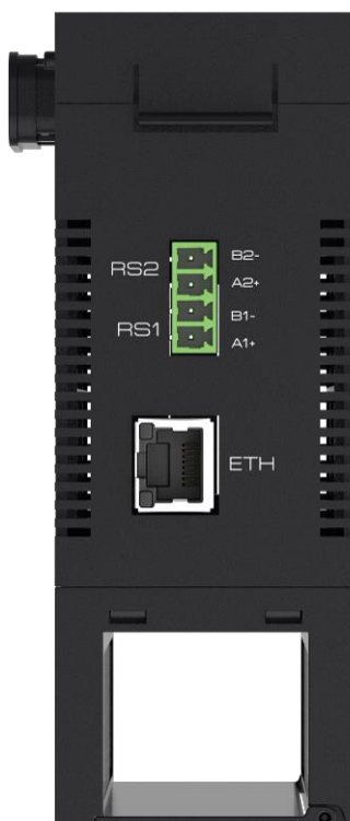
Рисунок 1.3 – Верхняя сторона модуля контроллера Simbol-300 S-300-DO16, S-300-DO32 с разъёмами интерфейсов
