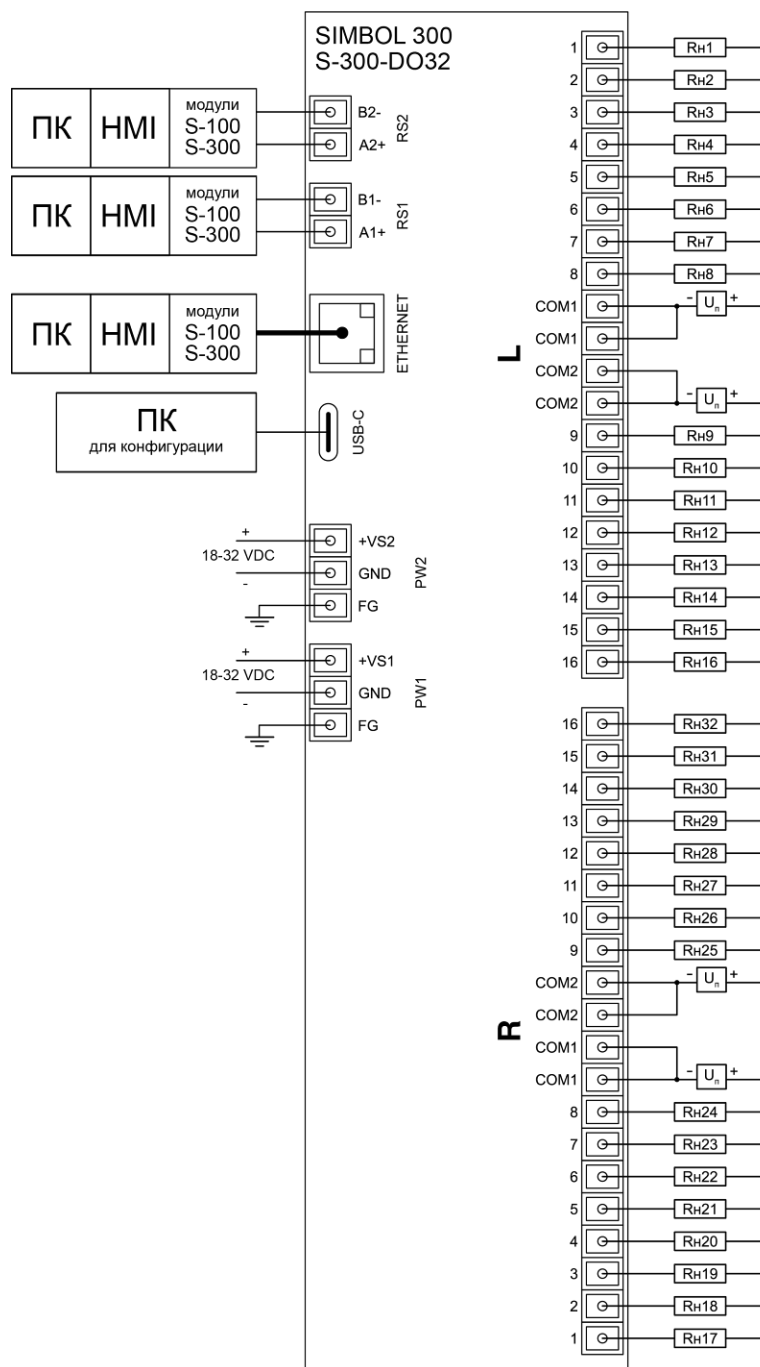
Рисунок 1.5 – Схема подключения модуля контроллера Simbol-300 S-300- DO32, S-300-DO16
