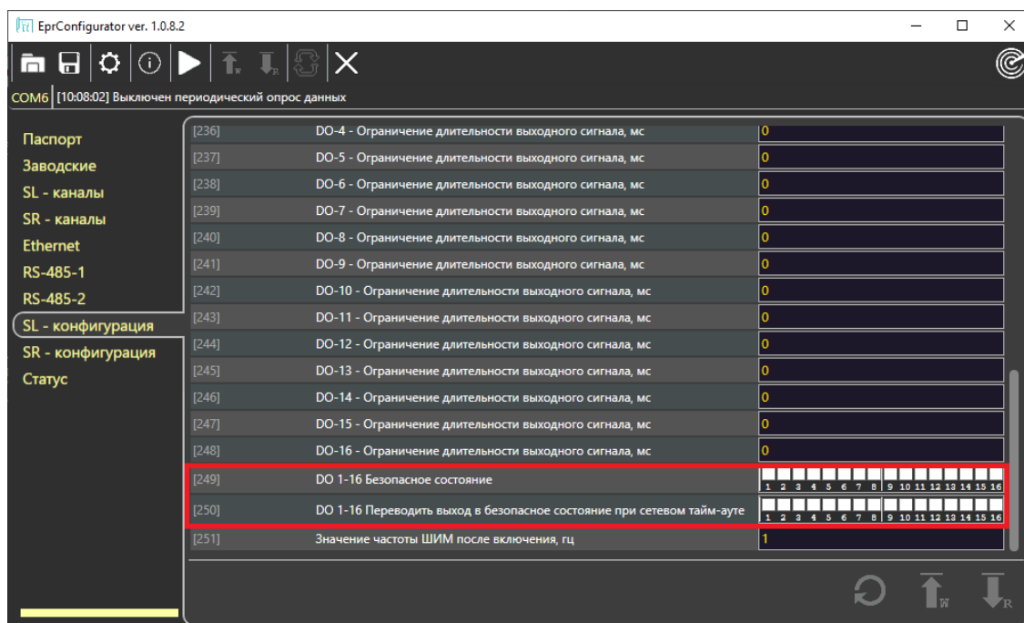
Рисунок 1.6 – Настройка безопасного состояние модуля контроллера Simbol-300 S-300-DO16, S-300-DO32 в СПО EprConfigurator
