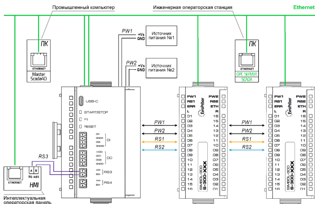
Рисунок 1.5.4.1 – Пример схемы подключения устройств к S-300-CPU, S-300-CPU-D
