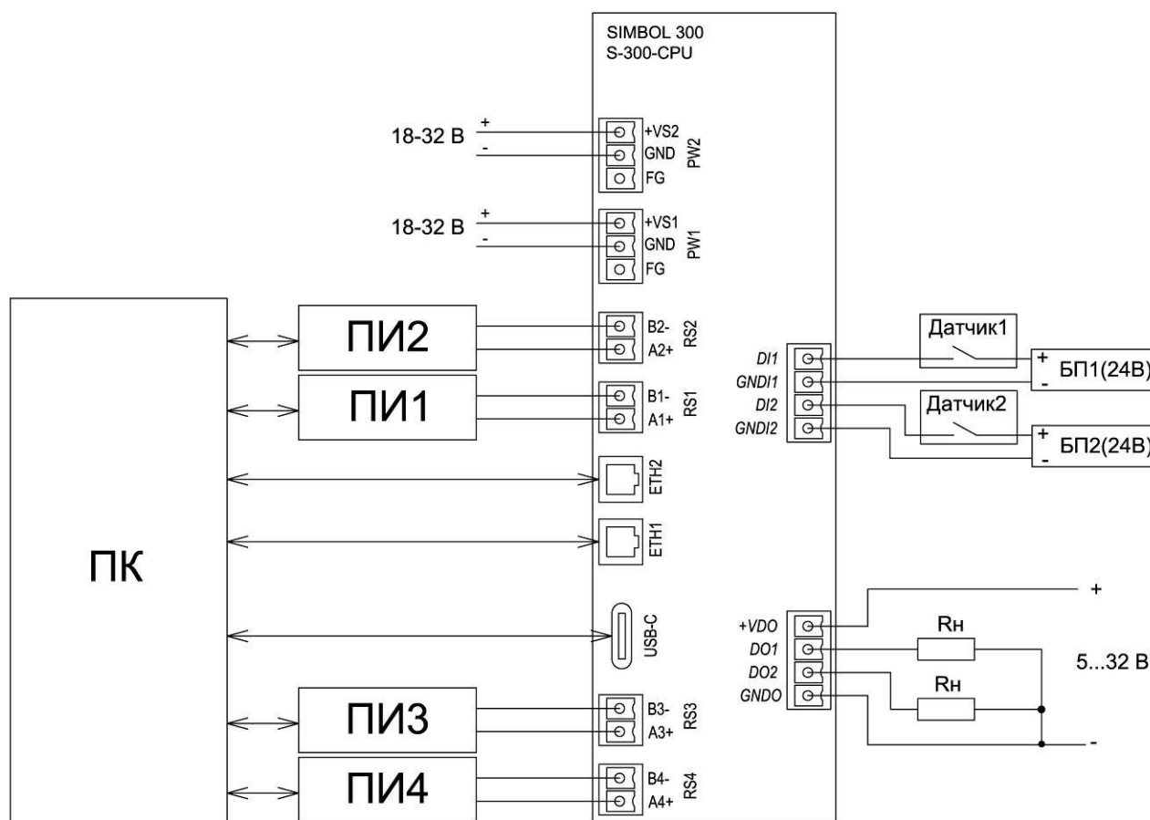
Рисунок 1.5.4.2 – Пример схемы подключения
