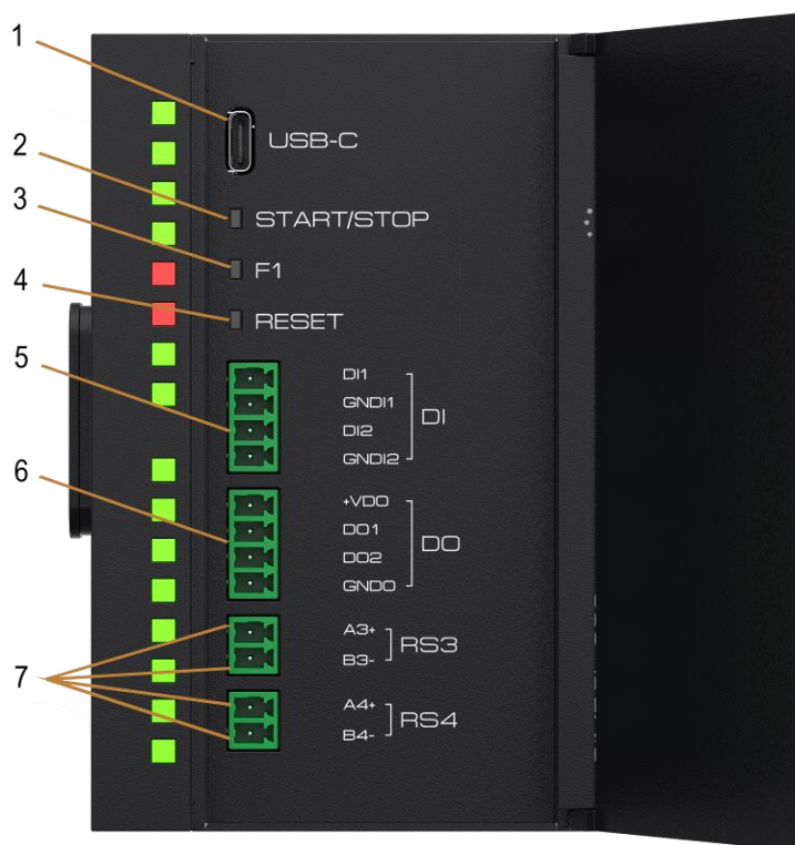
Рисунок 1.5.1.4 – Лицевая панель модулей S-300-CPU, S-300-CPU-D с открытой крышкой
