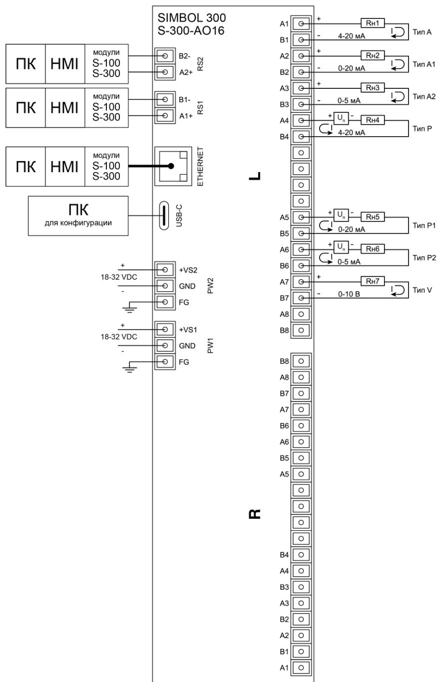
Рисунок 1.5 – Схема подключения модуля контроллера Simbol-300 S-300- AO16 (S-300-AO8)
