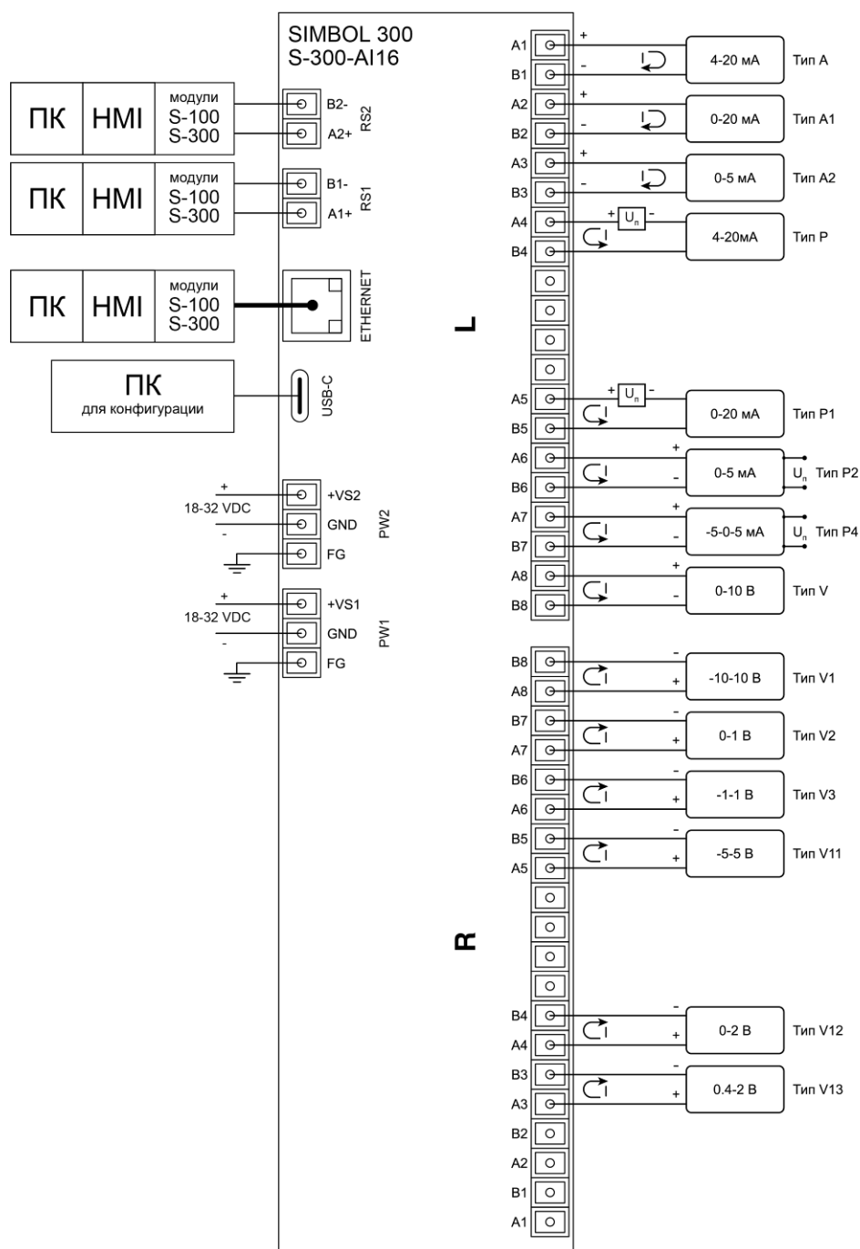
Рисунок 1.5 – Схема подключения модуля S-300- AI16 (S-300-AI8)
