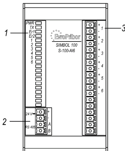
Рисунок 4.1 – Лицевая панель модуля S-100-A16
