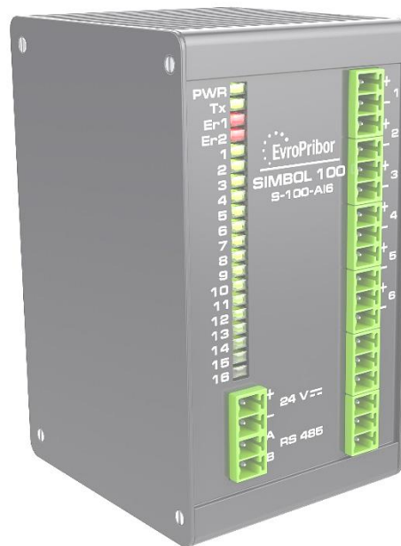
Рисунок 3.1 – Внешний вид модуля S-100-A16
