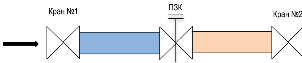
Рисунок 1 – Линия редуцирования с указанием рабочих объемов
