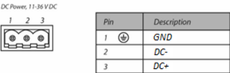
Рисунок 9 – Подключение электропитания к панели оператора
