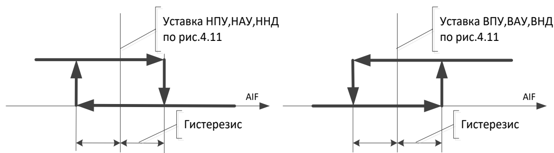
Рисунок 8 – Гистерезис
