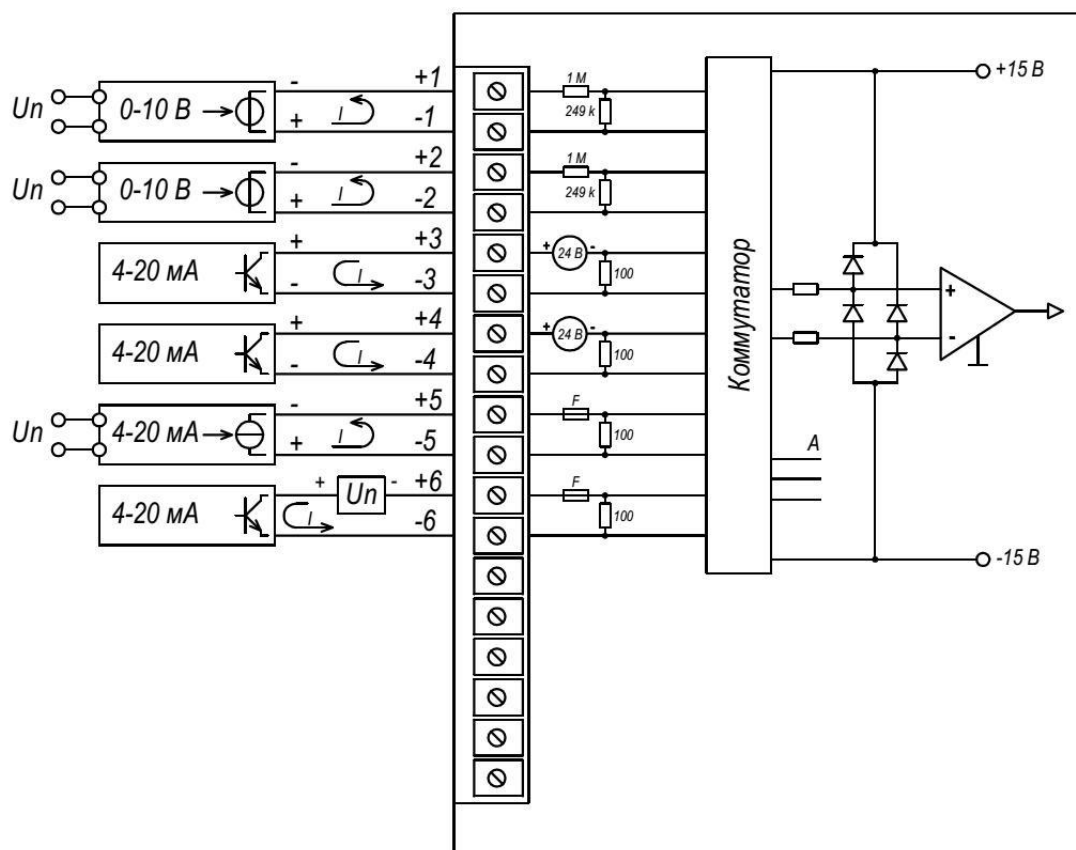
Рисунок 13 – Примеры схем подключения ПП различного типа к модулю контроллера измерительного Simbol-100-AI6
