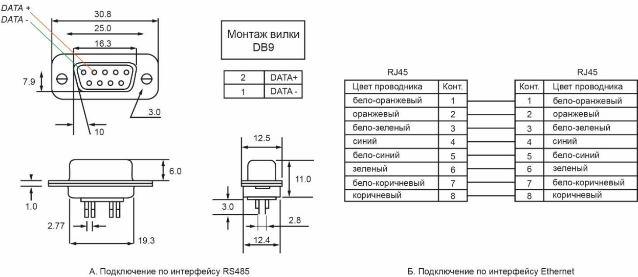
Рисунок 11 – Подключение интерфейсов RS485 и Ethernet к панели оператора
