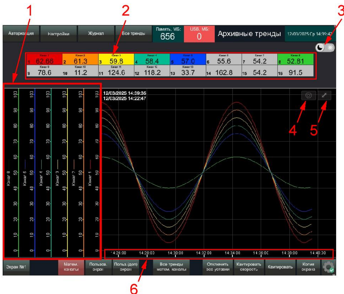
Рисунок 87 – Окно «Все тренды»
