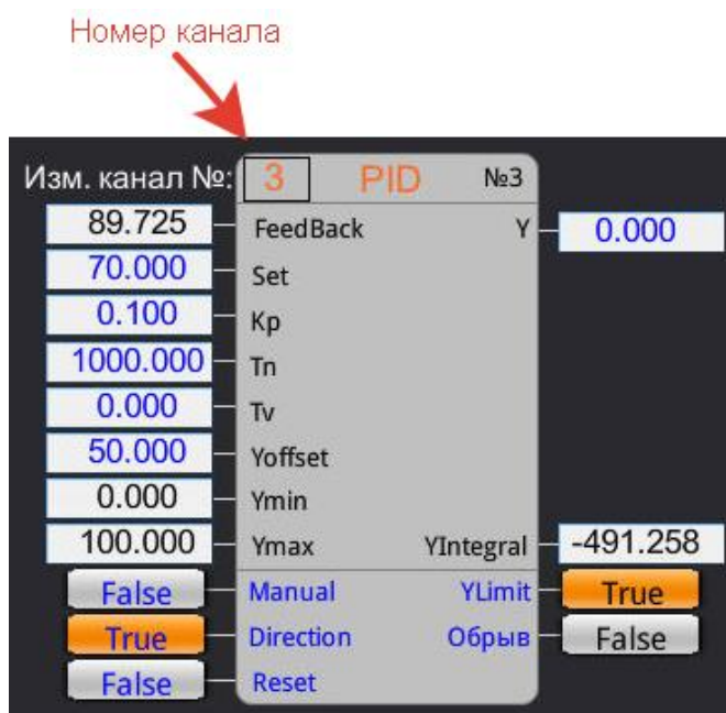
Рисунок 80 – Подключение ПИД-регулятора к выбранному каналу
