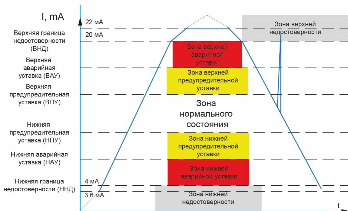
Рисунок 7 – Уставки и их зоны
