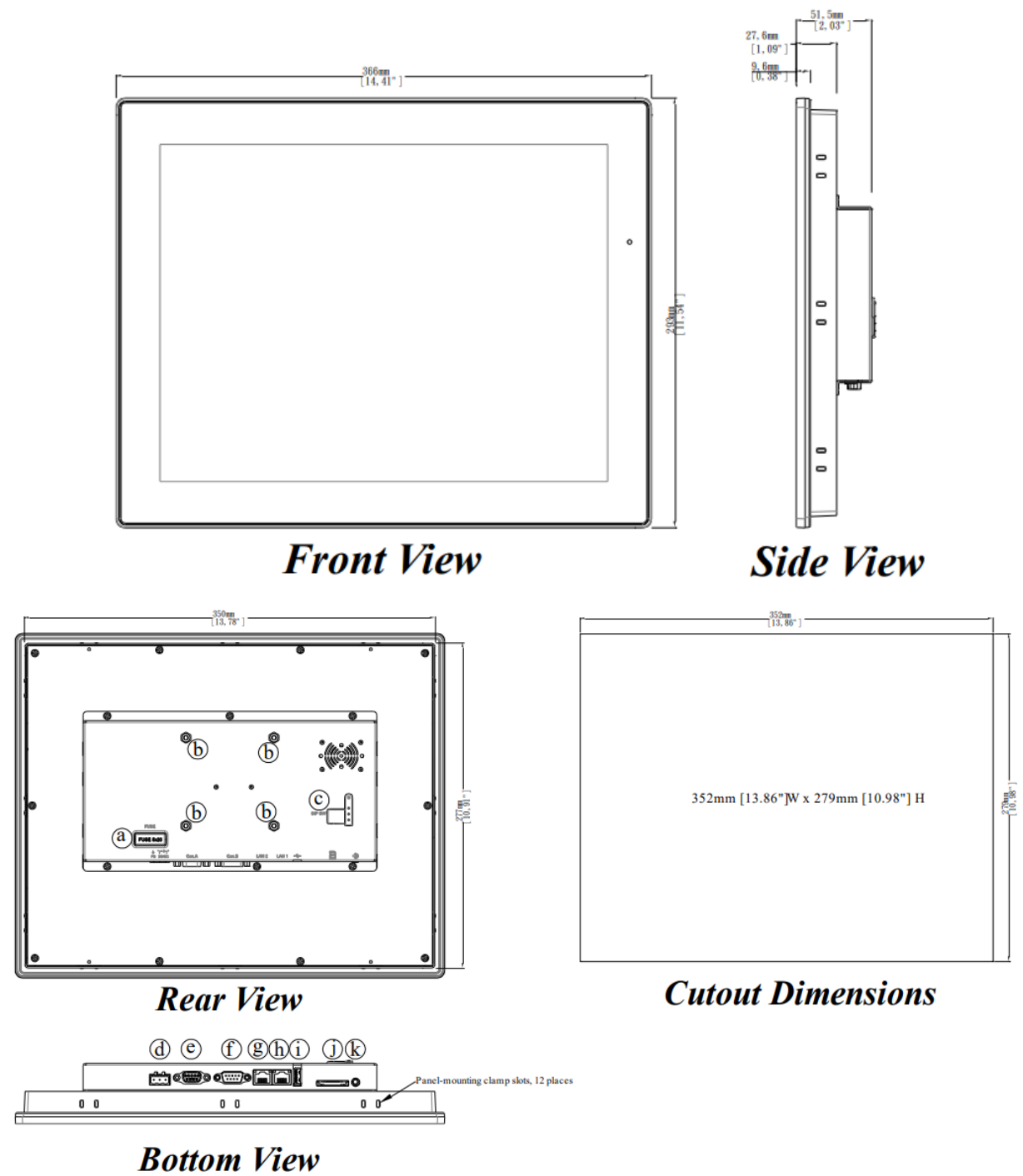
Рисунок 3 – Габаритные и установочные размеры панели cMT3152XV2(15'')
