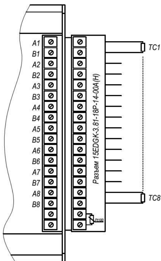
Рисунок 15 – Схема подключения термодатчиков к модулю Simbol-100- TC8
