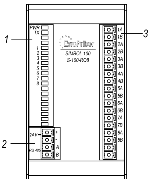
Рисунок 1.2 – Лицевая панель модуля релейных выходов S-100-RO8
