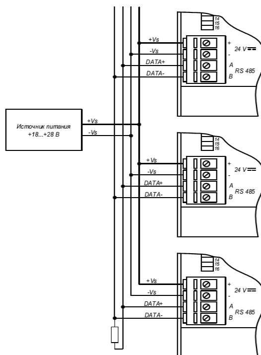
Рисунок 1.5 – Подключение модулей к информационной сети
