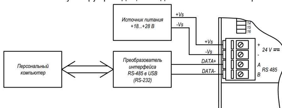
Рисунок 1.4 – Подключение модулей к порту ПК
