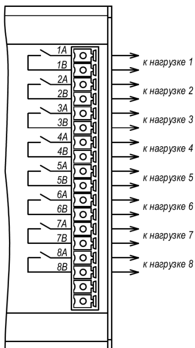
Рисунок 1.3 – Контактные группы модуля S-100-RO8
