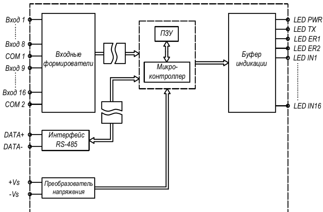
Рисунок 1.3 – Функциональная схема модуля S-100-DI16
