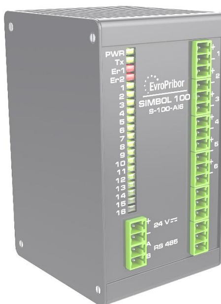
Рисунок 3.1 – Внешний вид модуля S-100-AI6
