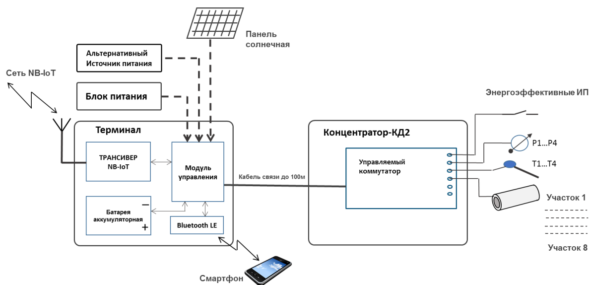
Рисунок 1 – Структура ПТК REGION-telematic/PTC
